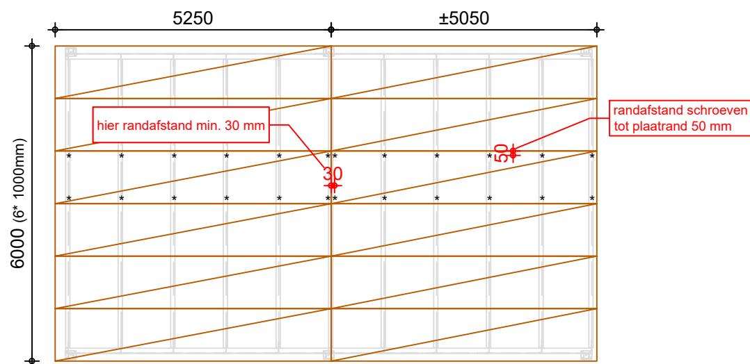
LEGPLAN VLOERPLATEN 12 stuks Vloerplaat 5.250x1.000x38 mm
